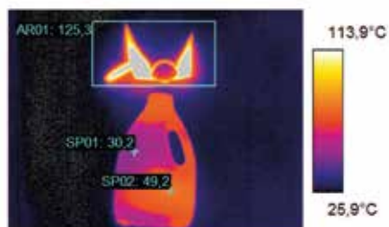
Infrarosso di uno stampo soffiaggio in acciaio + alluminio
